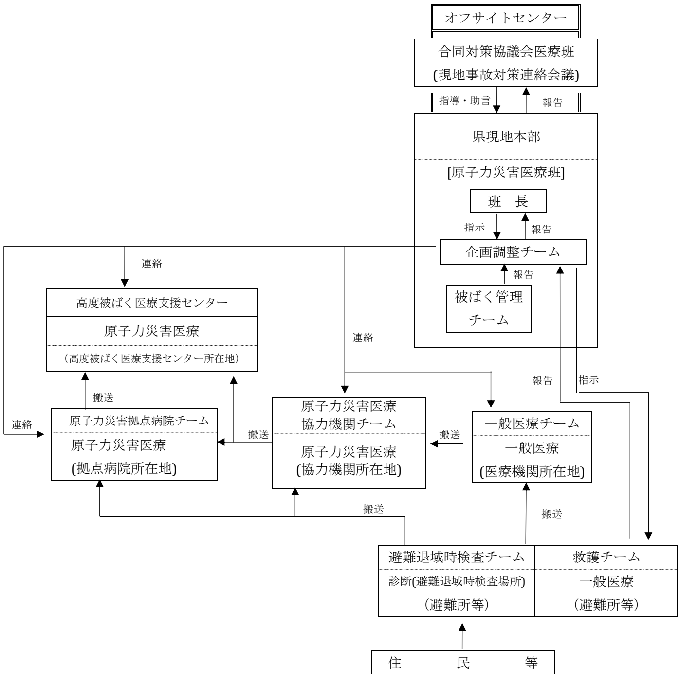
原子力災害医療措置系統図
